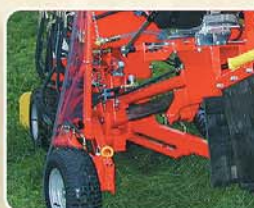
Ruote frontali regolabili in larghezza Roues frontales réglables en largeur
